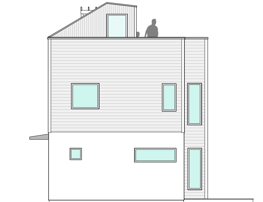
Fasade Vest
